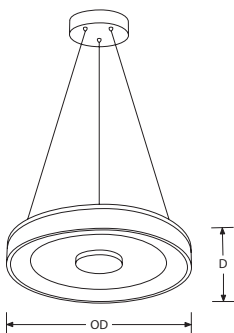
AA-PD32018 (OD) 320mm Overall (Ø) (D) 64mm Depth
